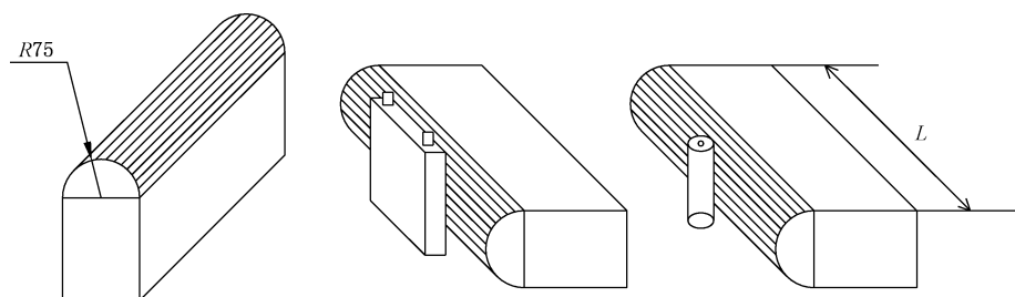
图 A.1 电池单体挤压板和挤压示意图
