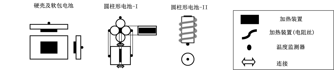
图 A.2 热失控试验加热示意图
