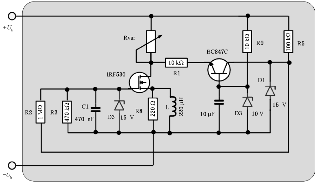
图 B.4 Power-i 模拟负载示例
