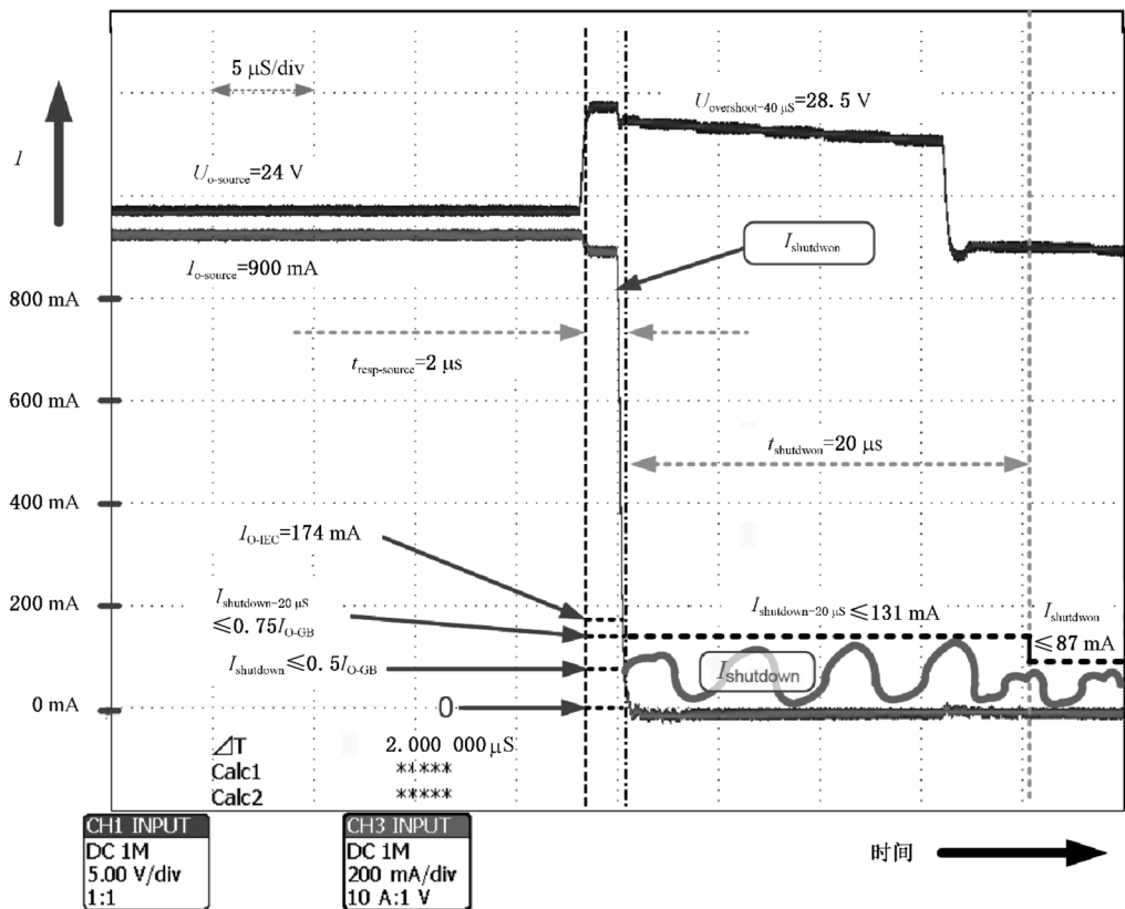
图 C.5 确定响应时间 t_{\text{resp-source}} 的示波图示例
