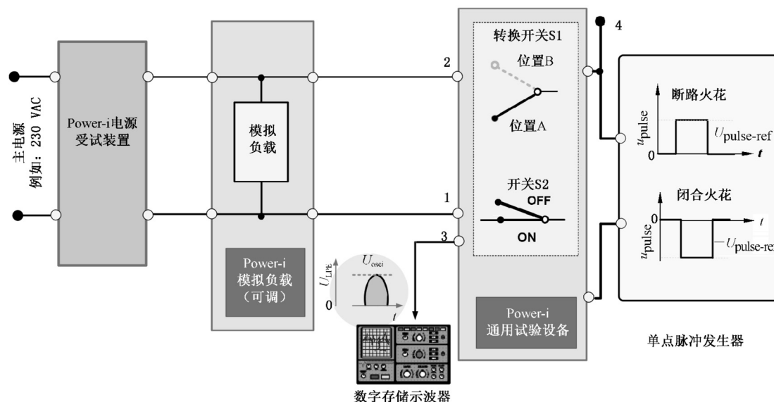
图 C.6 确定评定系数 AF_{\text{source}} 的试验设备(基本原理)
