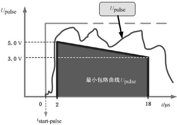
图 C.12 瞬态脉冲试验用试验脉冲 U_{\text{pulse}} 的评定参数
