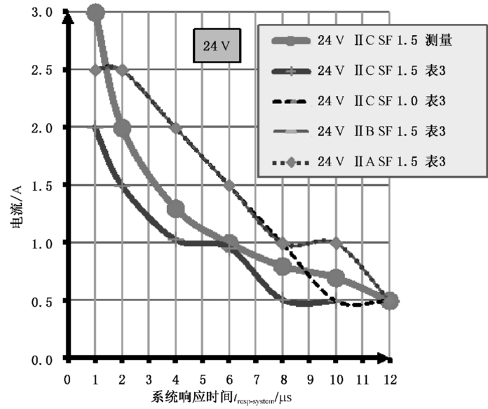
图 A.8 电压级别 24 V(24 VDC)的 Power-i 点燃曲线
