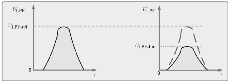
图 C.2 图 C.1 中端子 3 和 1 之间的脉冲输出
