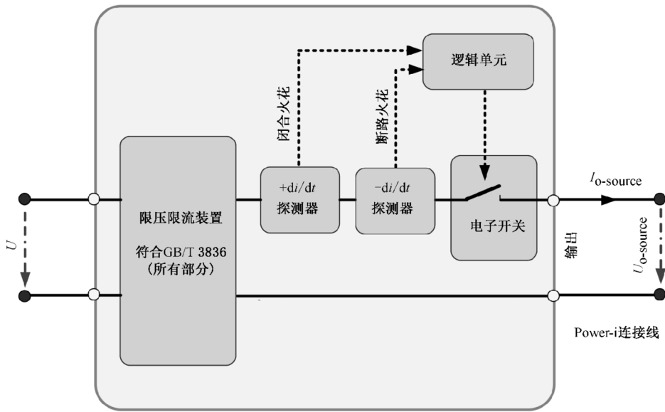
图 3 带限压限流装置的 Power-i 电源的元件
