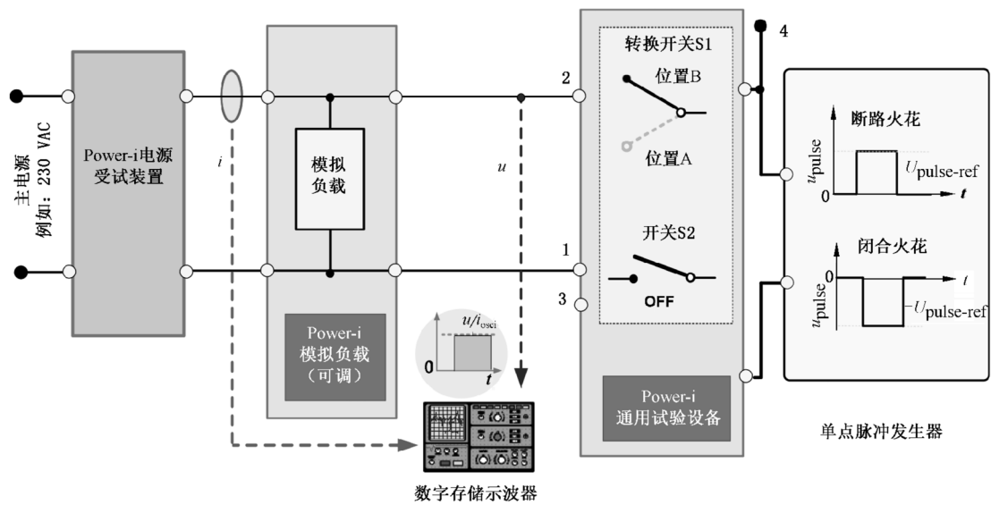
图 C.4 确定响应时间 t_{\text{resp-source}} 的设备基本原理
