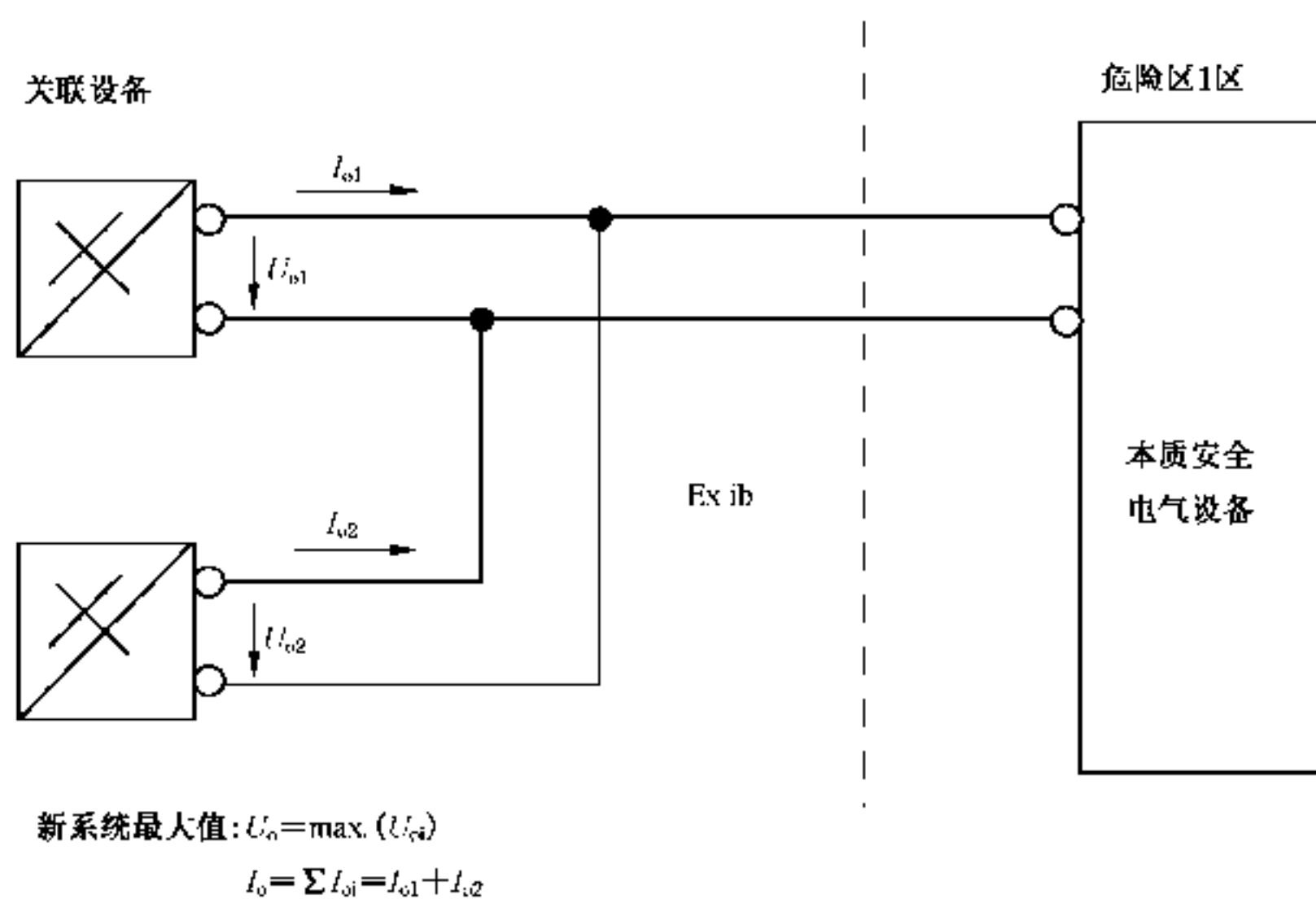
图 B.2 并联——电流相加
