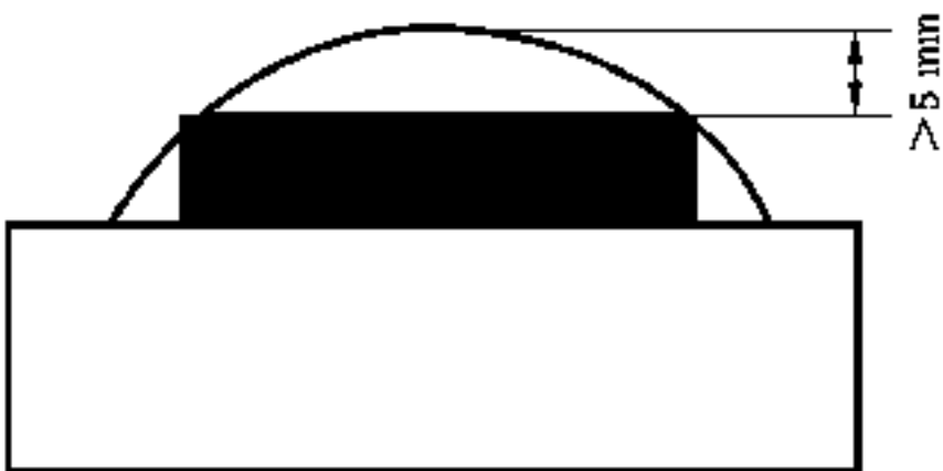
c) 设备侧面的超厚粉尘层
