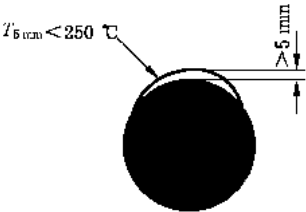
b) 设备顶部低点燃温度粉尘形成的超厚粉尘层
