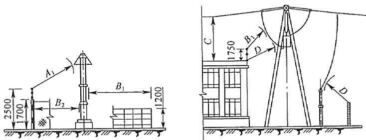
图 5.1.2-2 屋外 A_1 、 B_1 、 B_2 、 C 、 D 值校验
