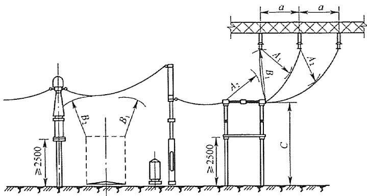
图 5.1.2-3 屋外 A_2 、 B_1 、 C 值校验
