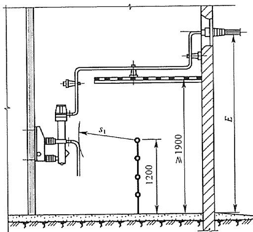
图 5.1.5-2 屋内 B_1 、 E 值校验
