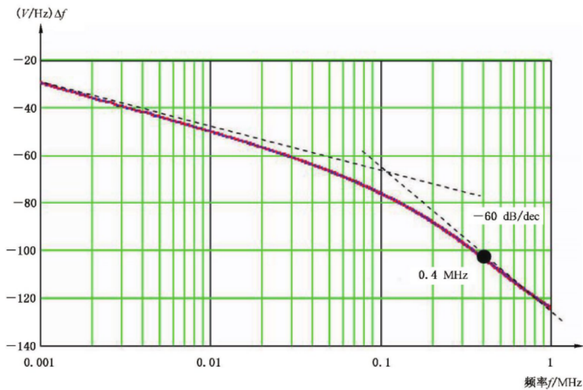
图 E.9 浪涌电压(10/700 μs):频域响应图, \Delta f = 0.2 \text{ kHz}
