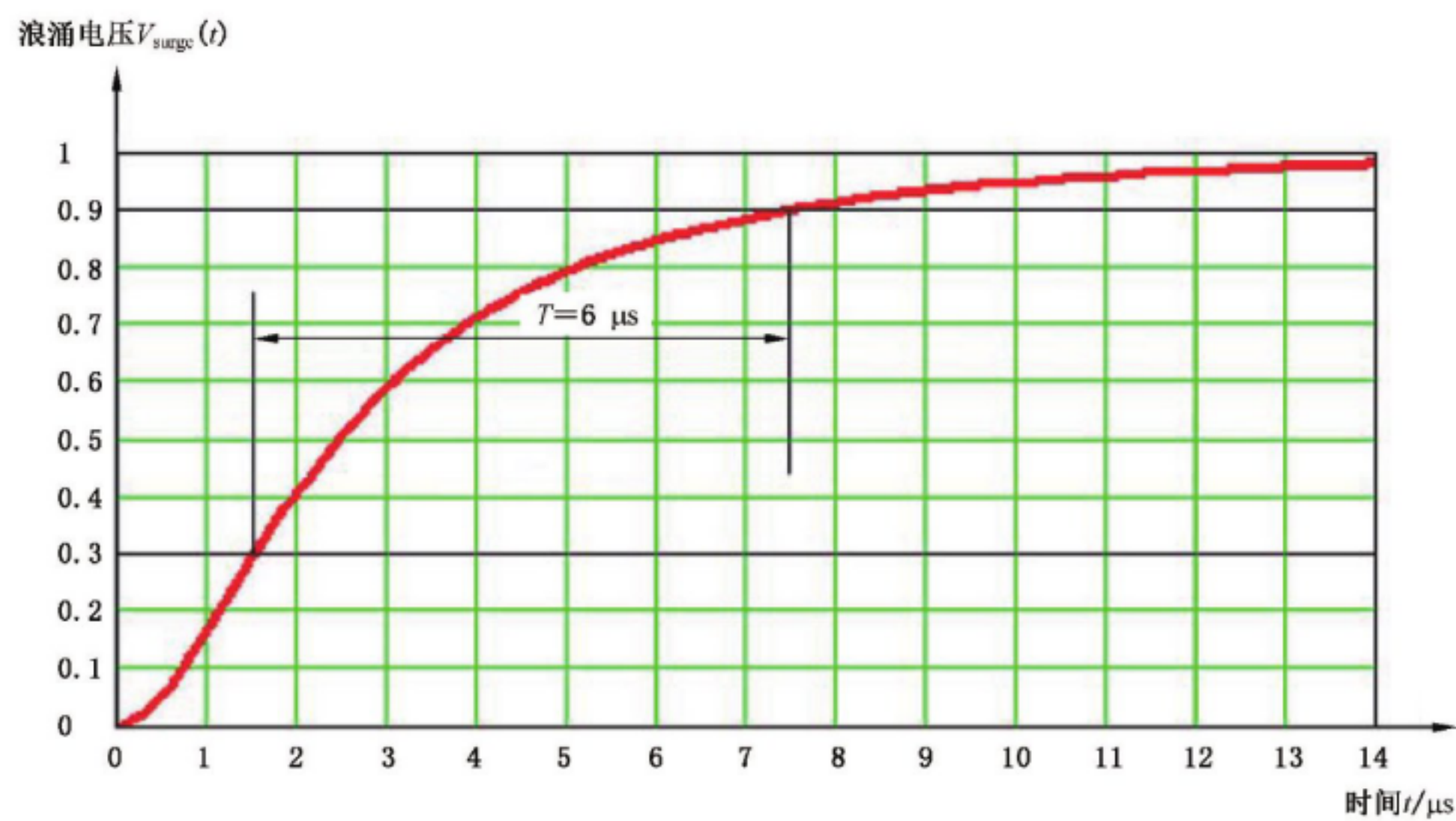
图 E.8 浪涌电压(10/700 μs):上升时间 T
