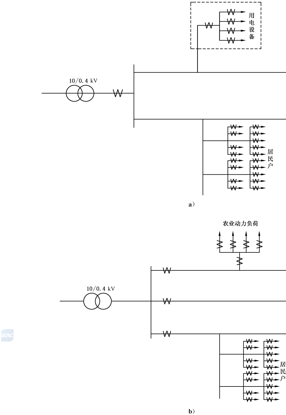
图 C.1 分级保护方式参考模式图
