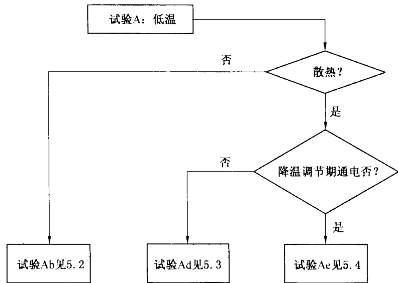
图 1 试验 A:低温试验方框图
