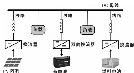
图 1 负荷接入公共直流母线的直流微网
