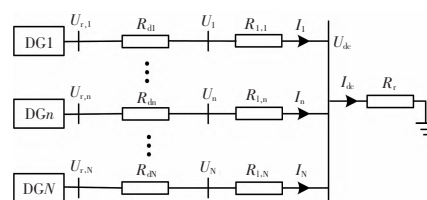
图 2 采用下垂控制的直流微网稳态等值电路
