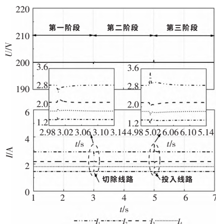
图 12 切除线路时的仿真结果
