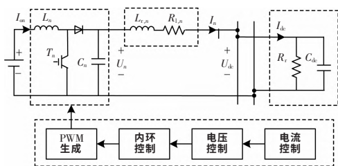
图 4 直流微网的暂态等值电路
