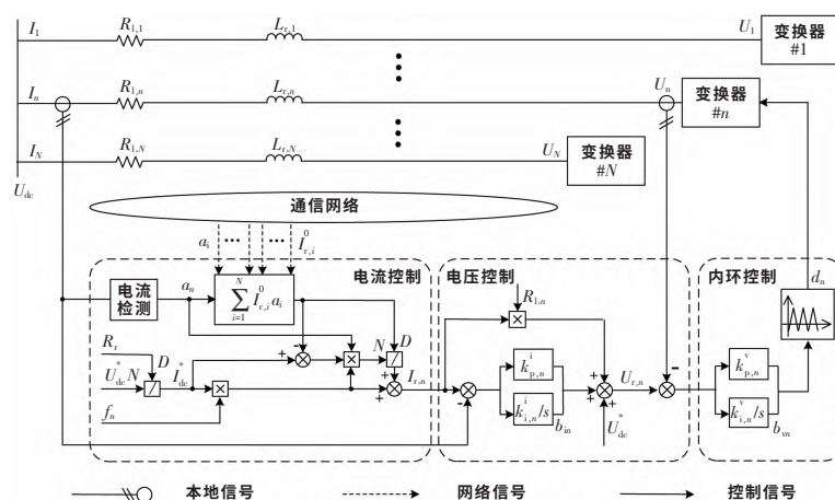
图 3 DG 单元的控制策略
