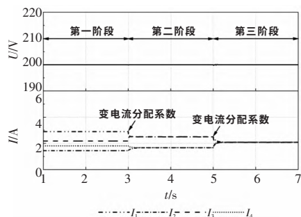
图 11 电流分配系数改变时的仿真结果
