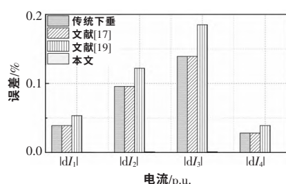
图 16 轻载时的电流相对误差
