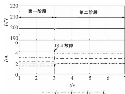
图 13 DG4 故障时的仿真结果
