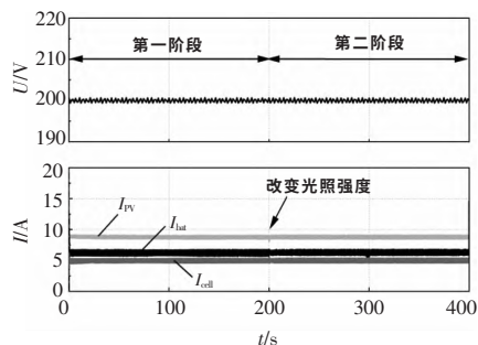
图6 光照强度改变时的仿真结果
