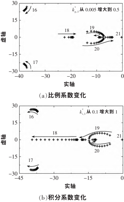
图 14 电压环 PI 参数变化时的根轨迹
