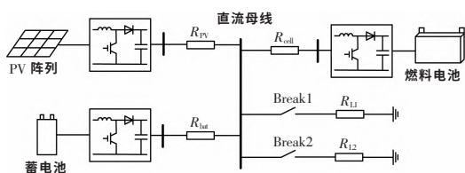
图5 光储直流微网系统结构示意图
