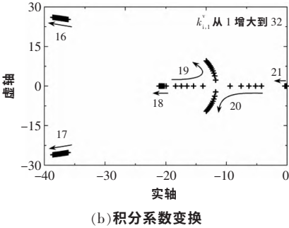
图 15 电流环 PI 参数变化时的根轨迹
