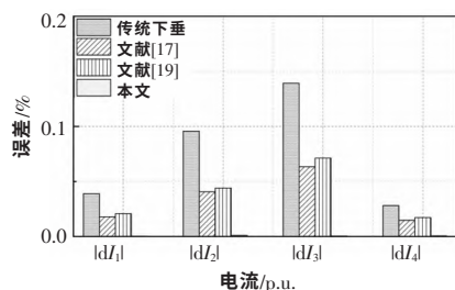
图 17 重载时的电流相对误差
