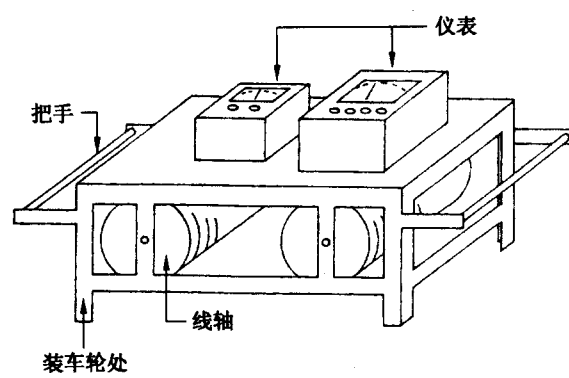
图 21 测试小车
