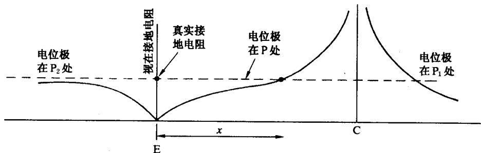
图 7 各种间距 x 时的视在接地电阻
