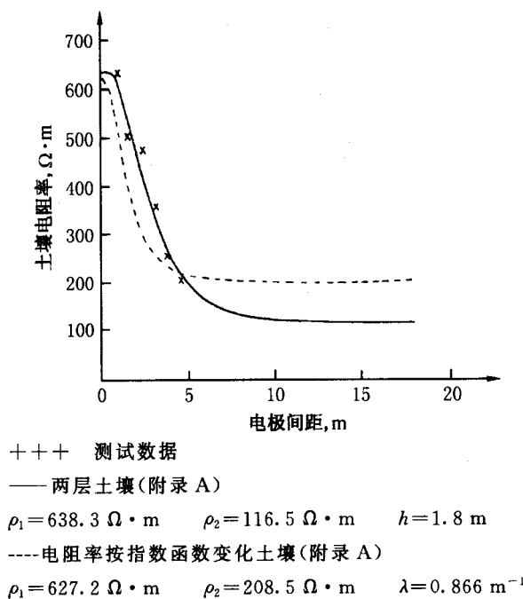
图 5 视在土壤电阻率与电极间距的关系实例
