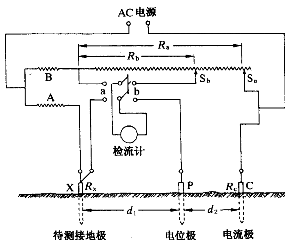
图 15 双平衡电桥
