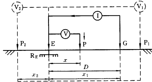
图 C1 电位降法
