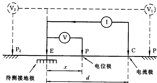
图 6 电位降法
