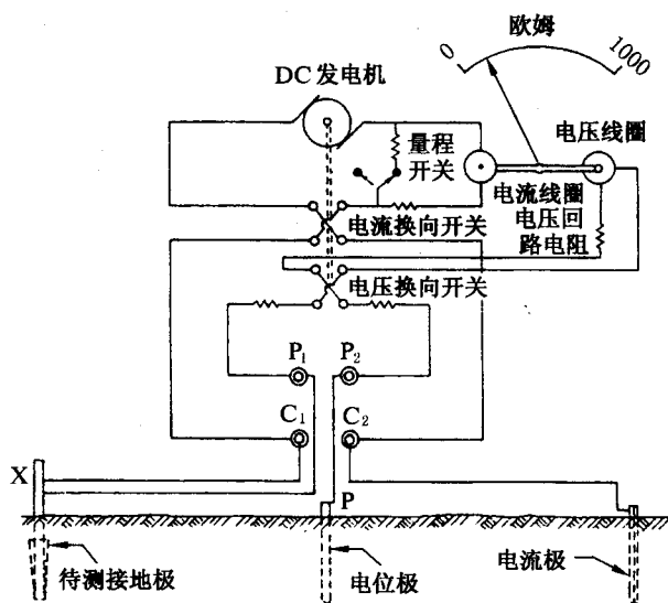
图 14 比率欧姆表
