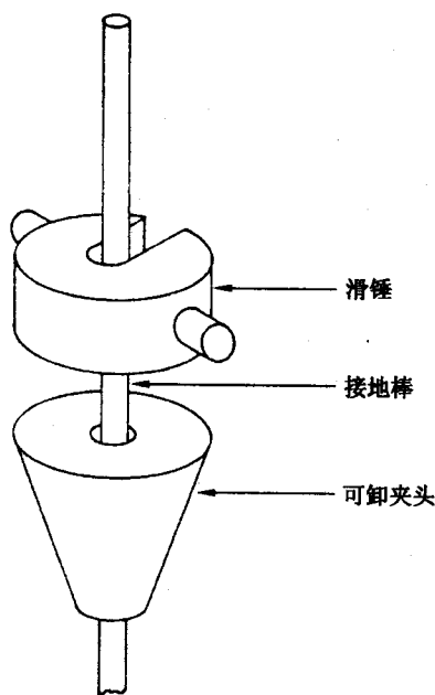
图 20 可卸夹头和滑锤
