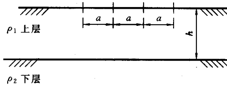
图 A1 两层土壤
