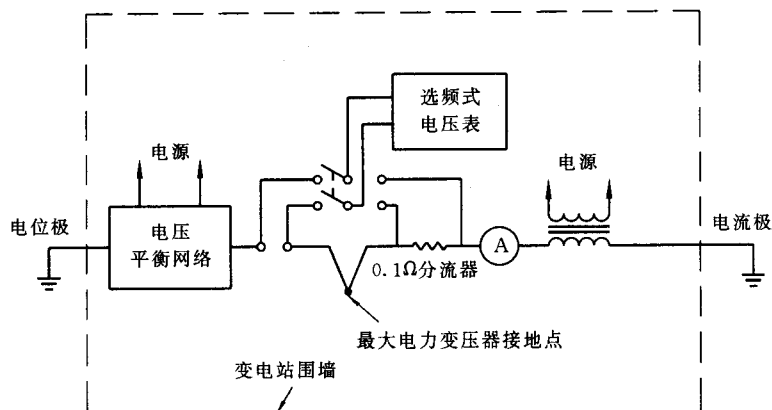
图 17 选频式电压表-电流表测量电路
