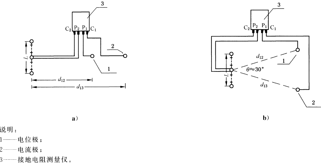
图 H.1 长接地体接地电阻测量接线图
