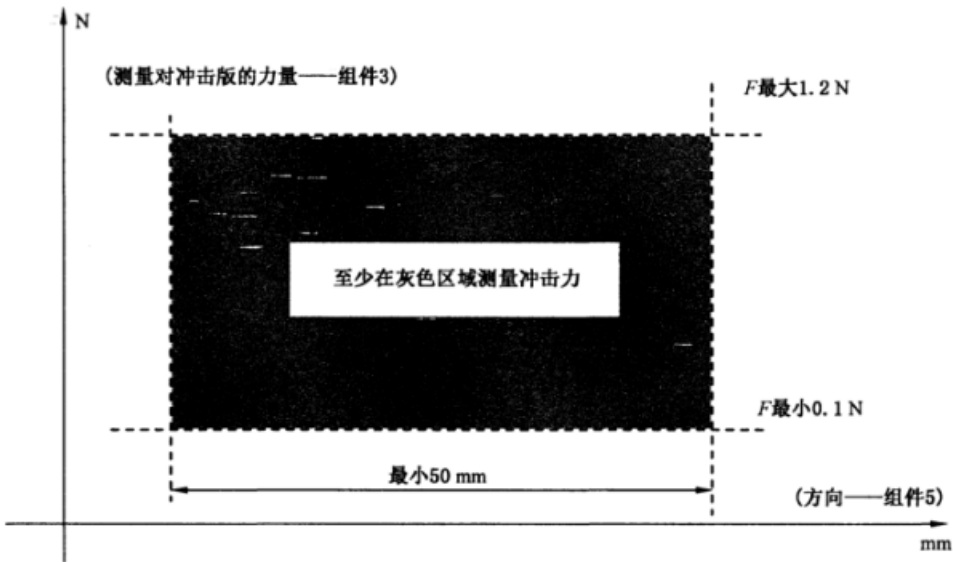
图 11 冲击力分布
