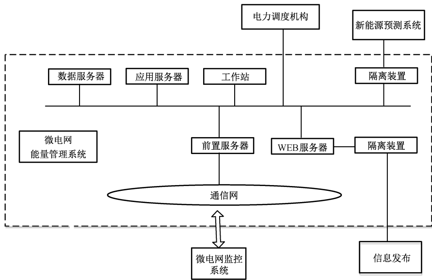
图 1 微电网能量管理系统结构与硬件配置
