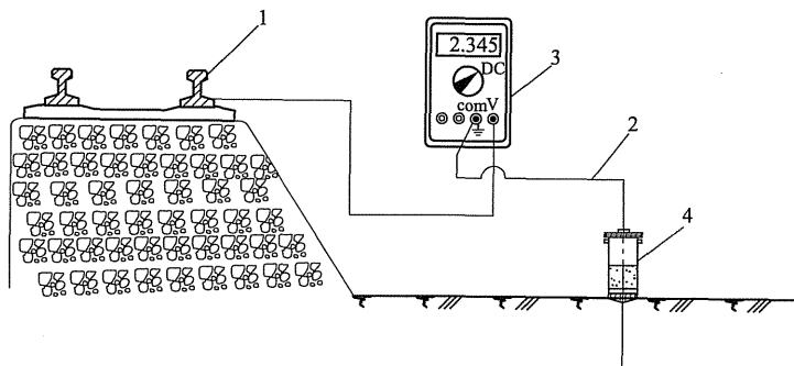
图 A.6.1 轨地电位测试接线图
