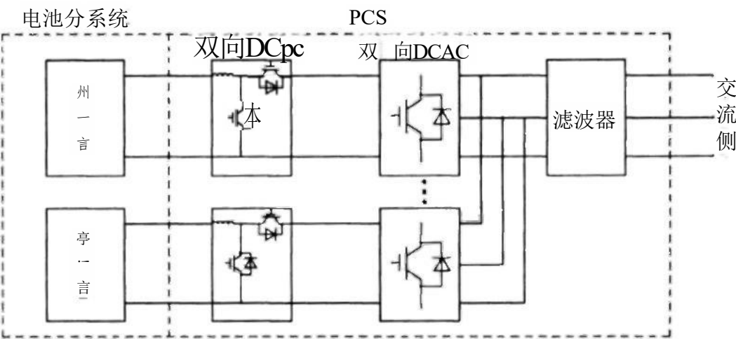
图 5 含 AC/DC 和 DC/DC 环节共交流侧的功率变换系统拓扑结构 (3)H 桥链式拓扑型。
