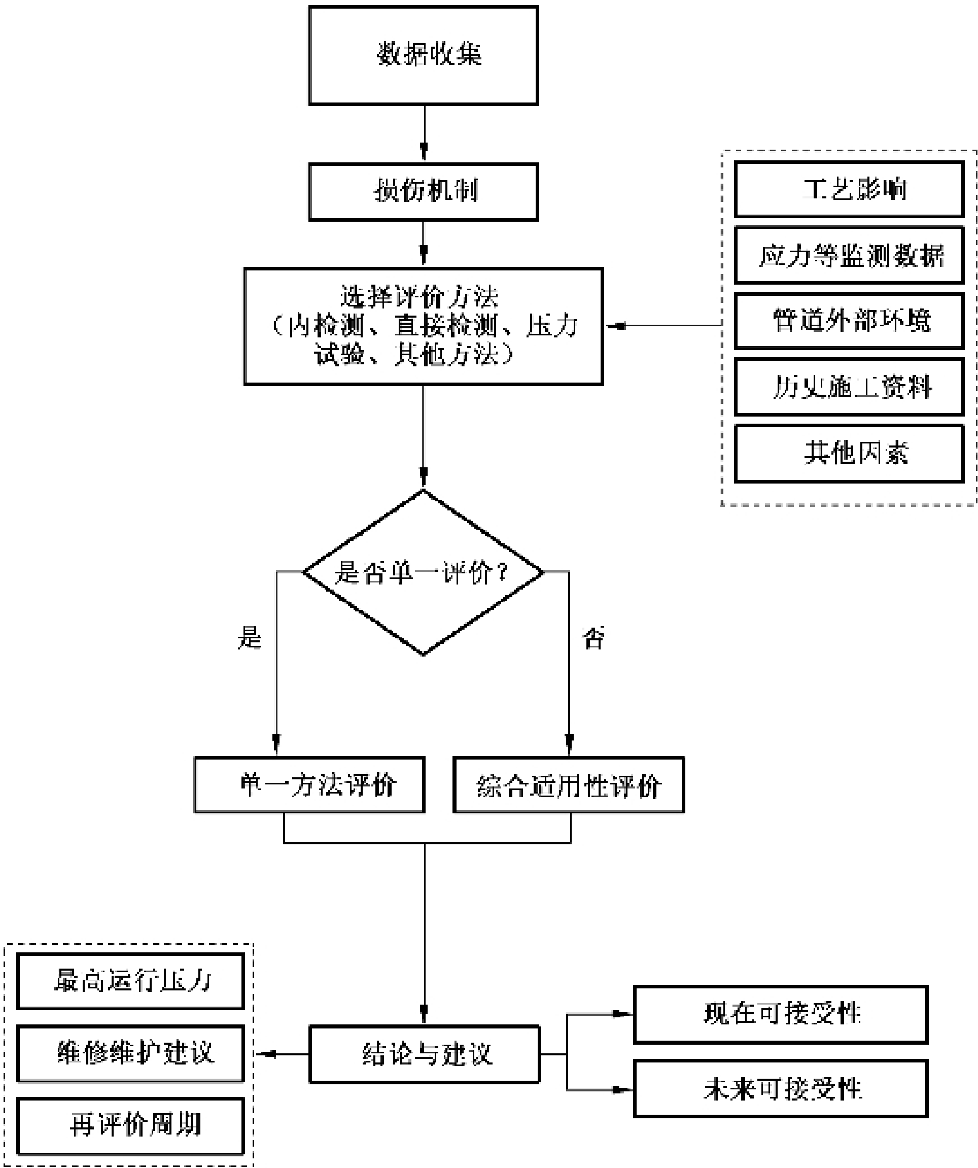
图 4 管道适用性评价流程
