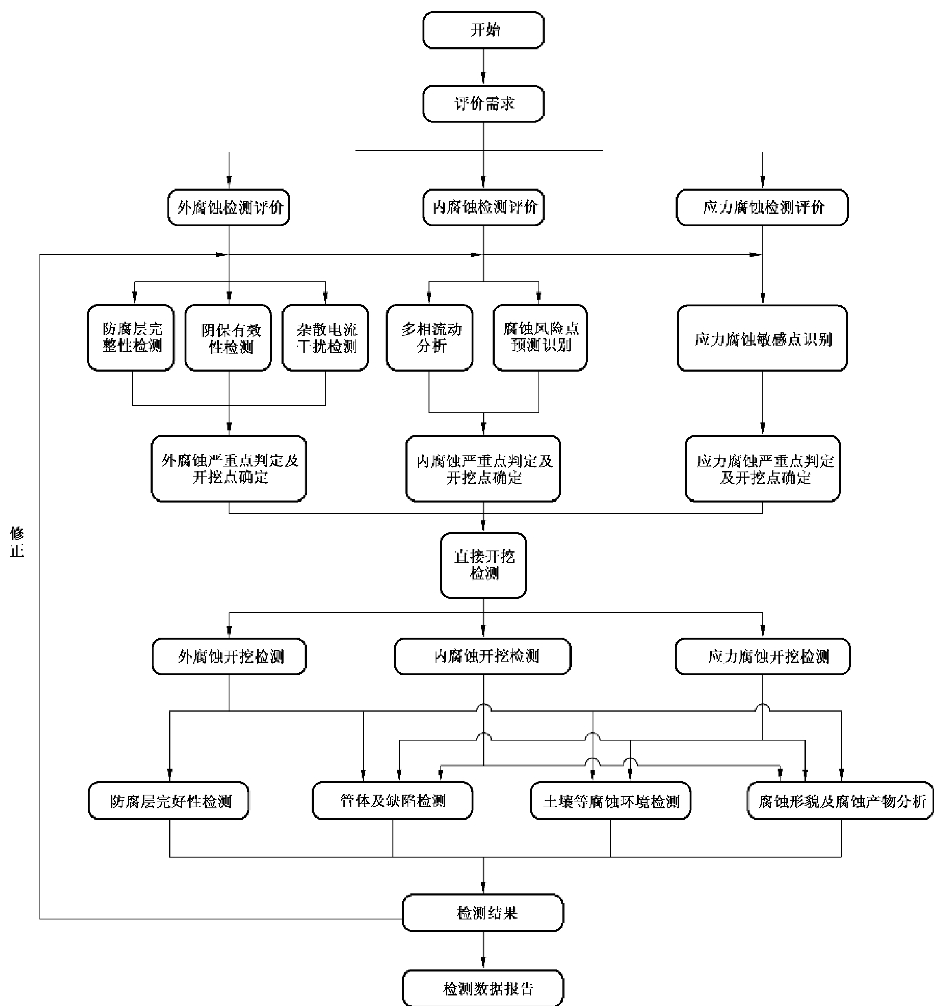
图3 直接检测流程图
