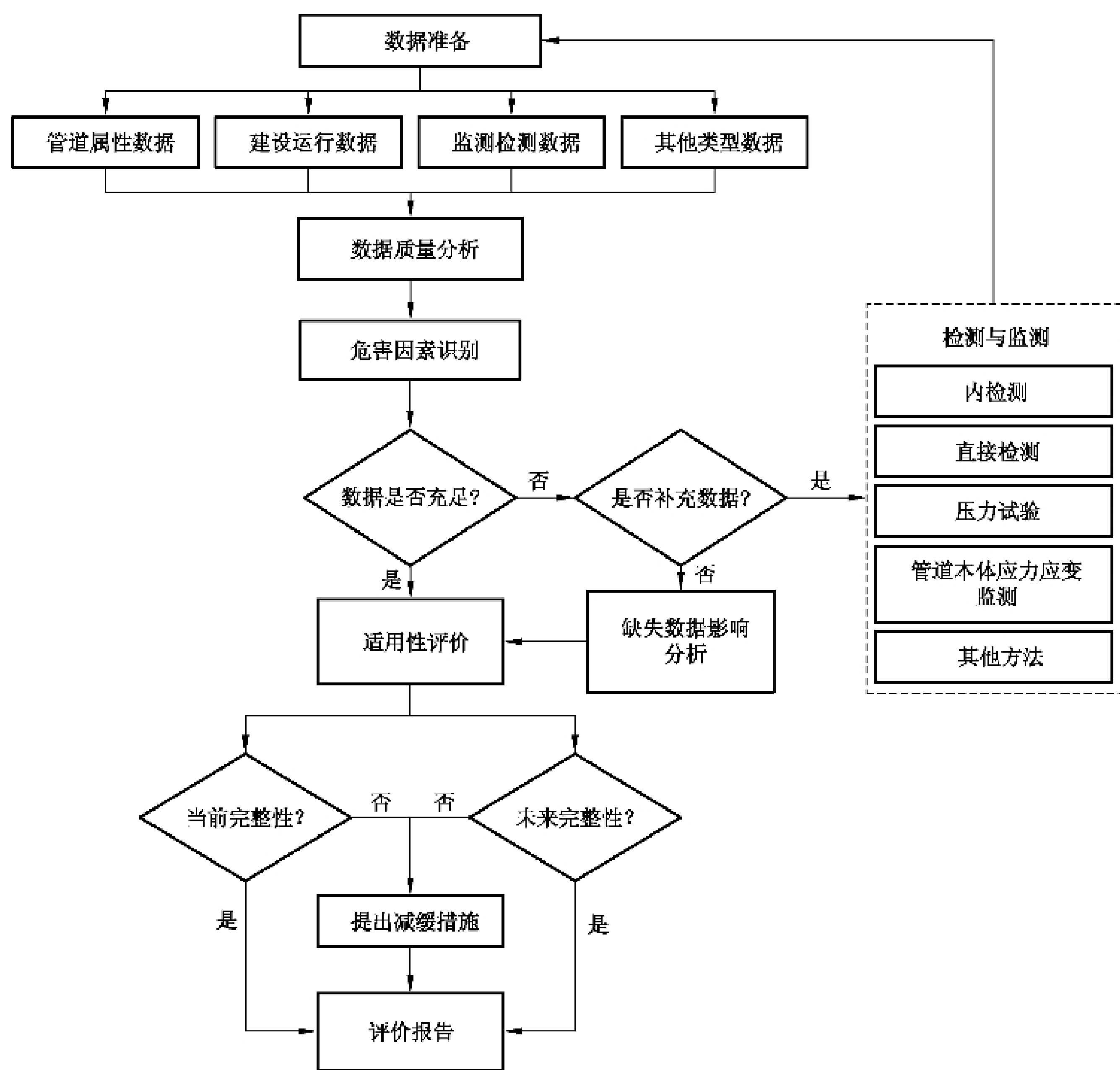
图 1 管道完整性评价工作流程
