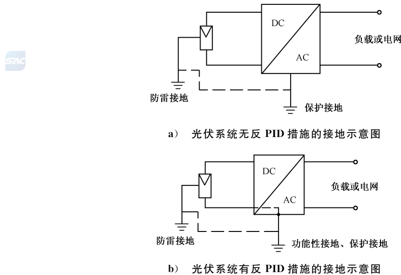
图 C.1 光伏发电系统接地示意图
