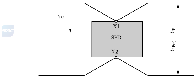
图 D.4 凯文接线方式示意图
