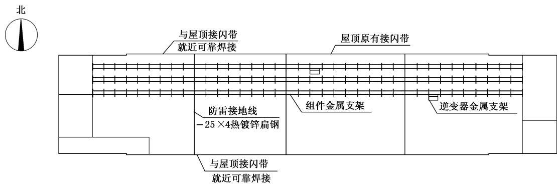
图 A.2 屋顶防雷平面示意图
