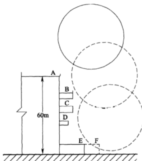
图 14 剖面示意
