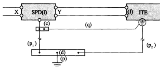
图 J. 2. 3-2 将多接线端子电涌保护器的有效电压保护水平减至最小所必需的安裝条件的例子
