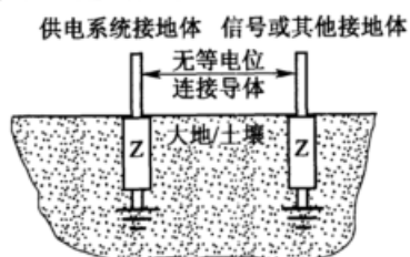
图 5 典型分开的接地
