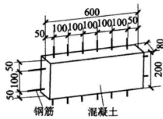
图9 试样的构造和尺寸
