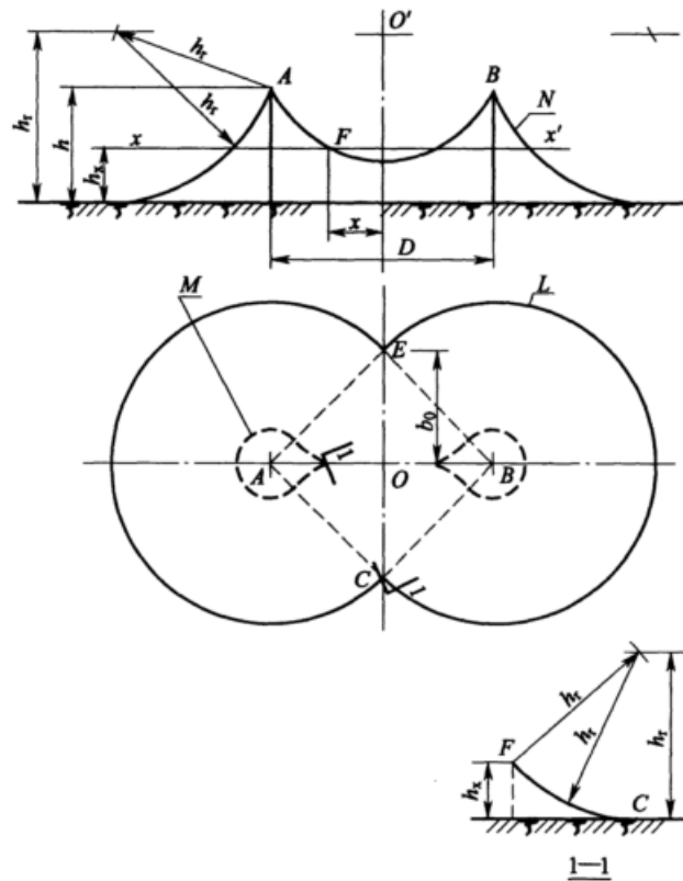
图 D.0.2 两支等高接闪杆的保护范围
