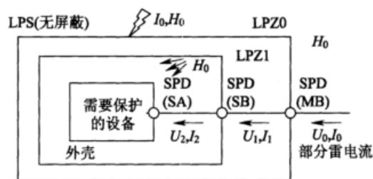
(d)仅采用协调配合好的电涌保护器保护 注：设备得到防线路导入电涌的保护， U_s 大大小于 U_0 和 I_s 大大小于 I_0 ， 但不需防 H_0 辐射磁场的保护。
