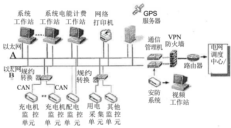
图 A 充电站监控系统结构示意图
