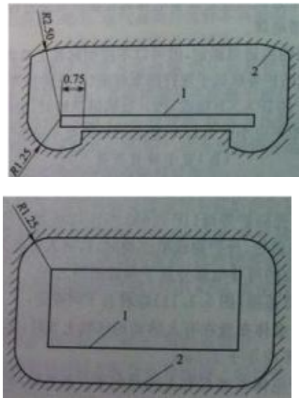
图5.1.11 伸臂范围(m) —平台；2—手臂可达到的界限
