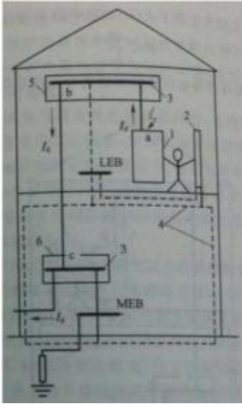
图3局部等电位联结的作用
