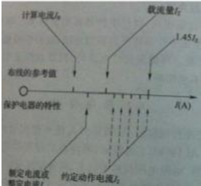
图7 过电荷保护电器的动力特性关系图
