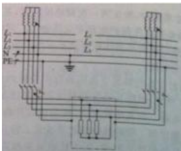
图2 在TN-S 系统中,采用具有断开中性极的开关可避免产生杂散电
