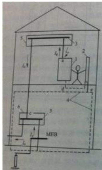
图4辅助等电位联结的作用
