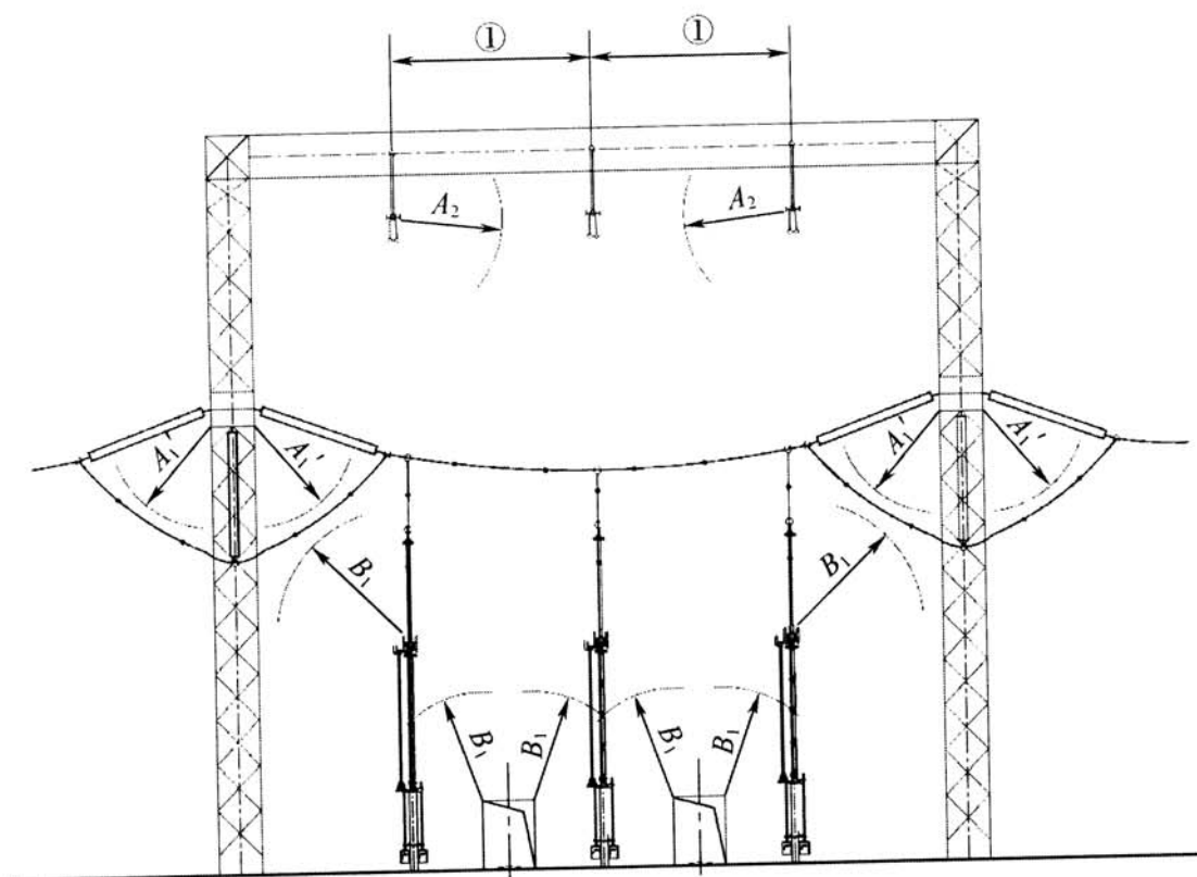
图 5.1.2-4 屋外 A'_1 、 A_2 、 B_1 值校验图
