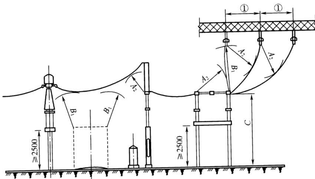
图 5.1.2-3 屋外 A_2 、 B_1 、 C 值校验图
