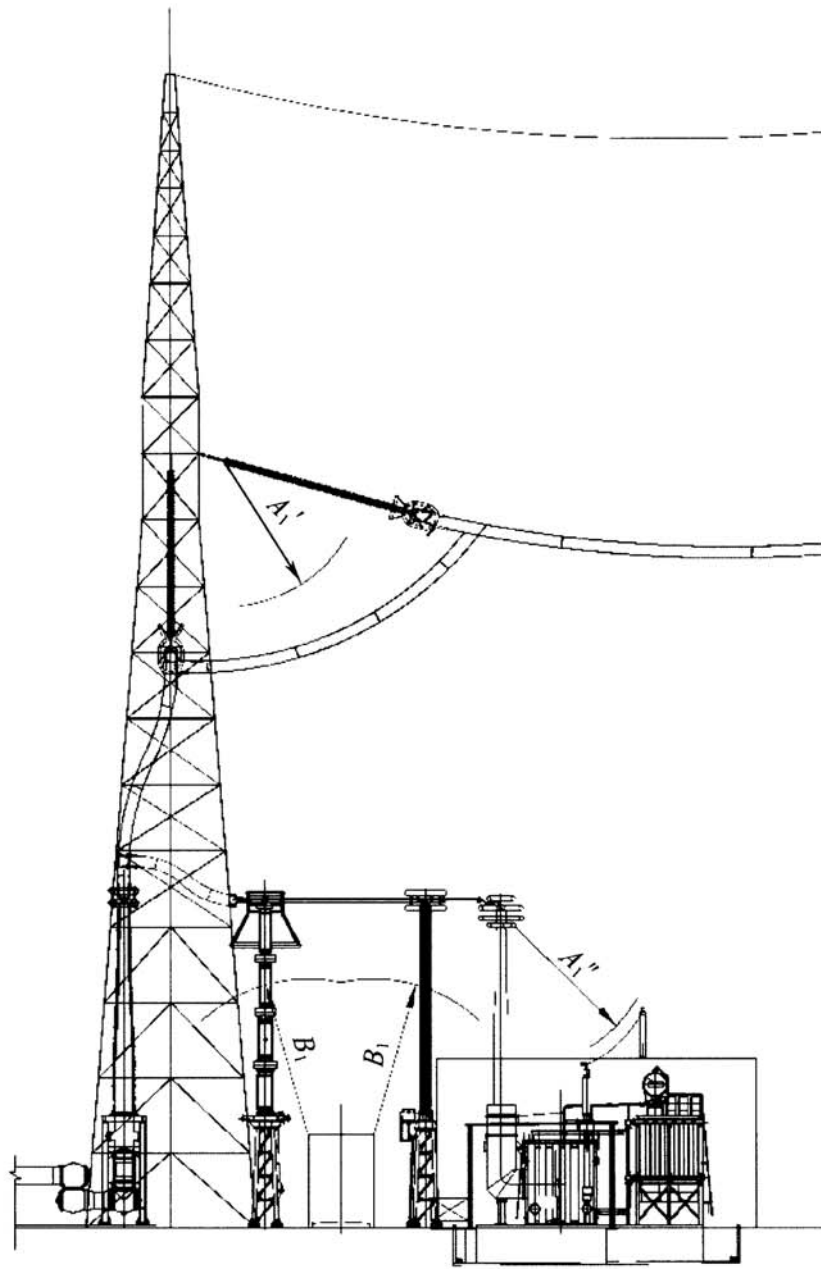
图 5.1.2-5 屋外 A'_1 、 A''_1 、 B_1 值校验图
