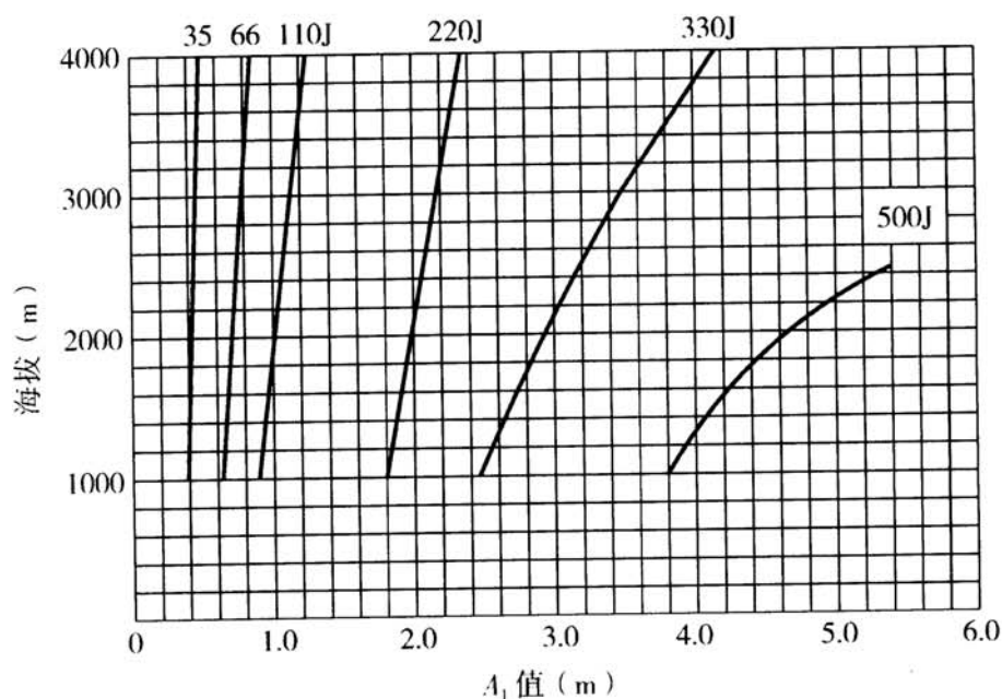
图 A.0.1 35kV~500kV 配电装置海拔大于 1000m 时 A 值的修正 注: A_2 值和屋内的 A_1 、 A_2 值可按本图之比例递增。
