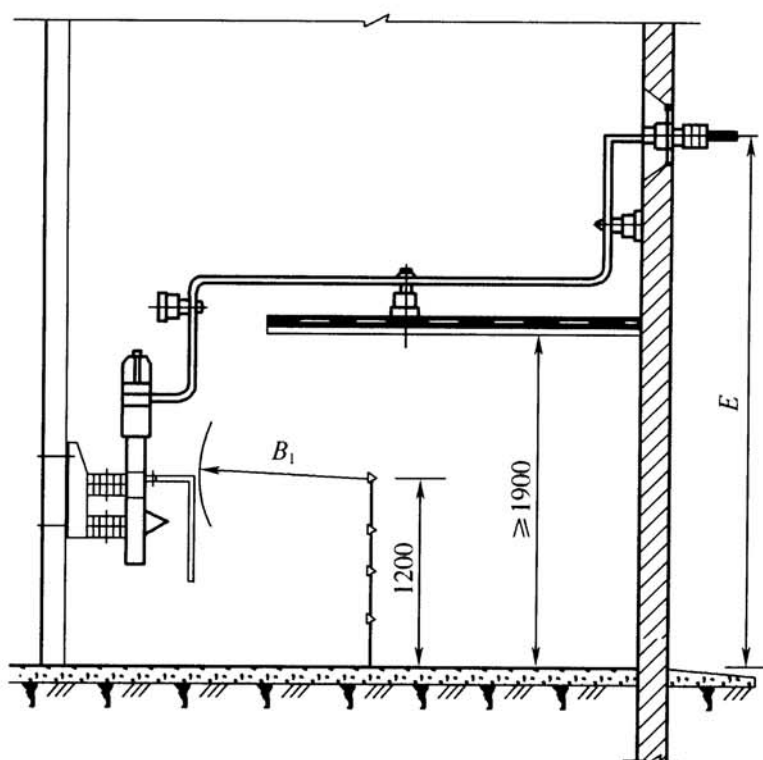
图 5.1.4-2 屋内 B_1 、 E 值校验图
