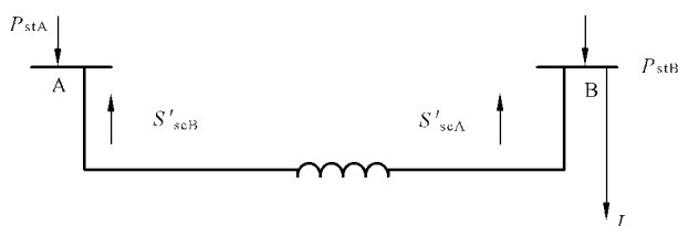
图 2 闪变传递计算示意
