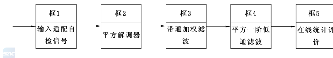
图 A.1 IEC 闪变仪模型的简化框图
