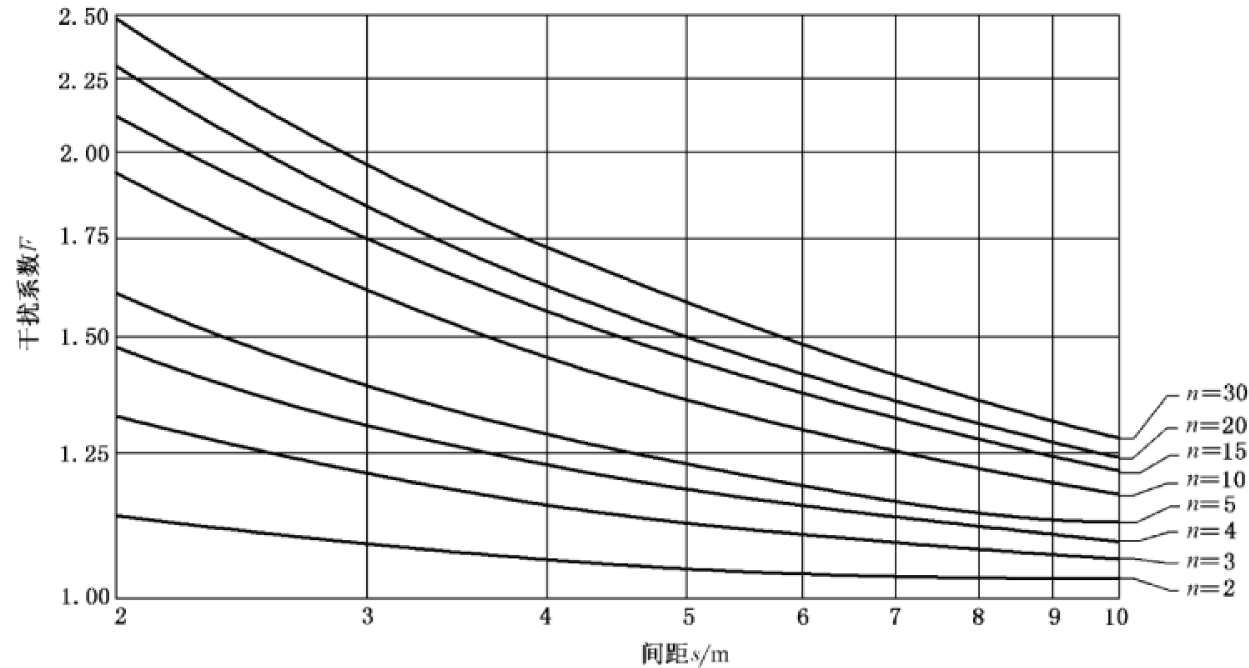
图 A.1 由 n 支阳极组成的阳极地床的干扰系数 F
