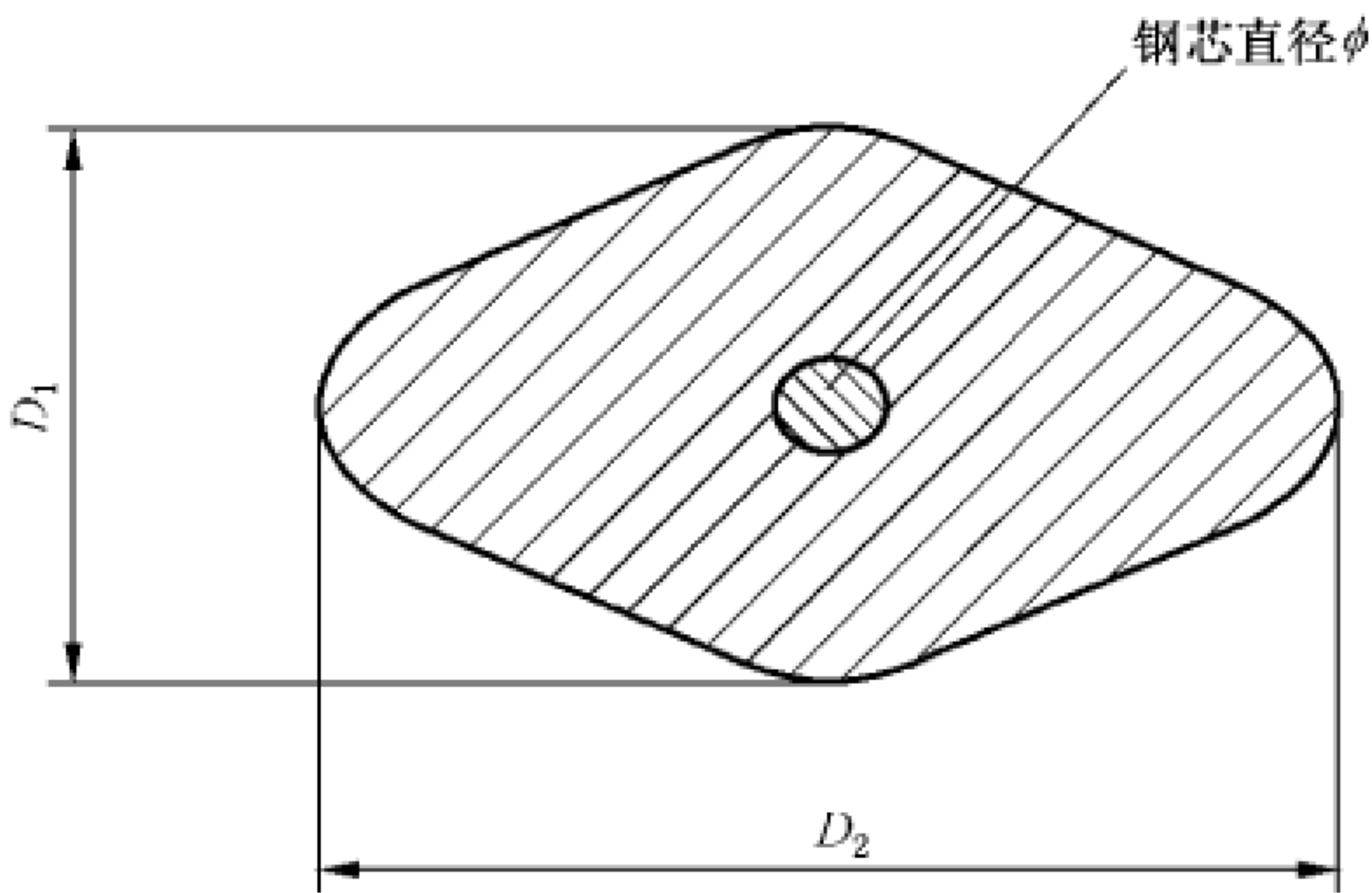
图 1 带状锌阳极的截面示意图
