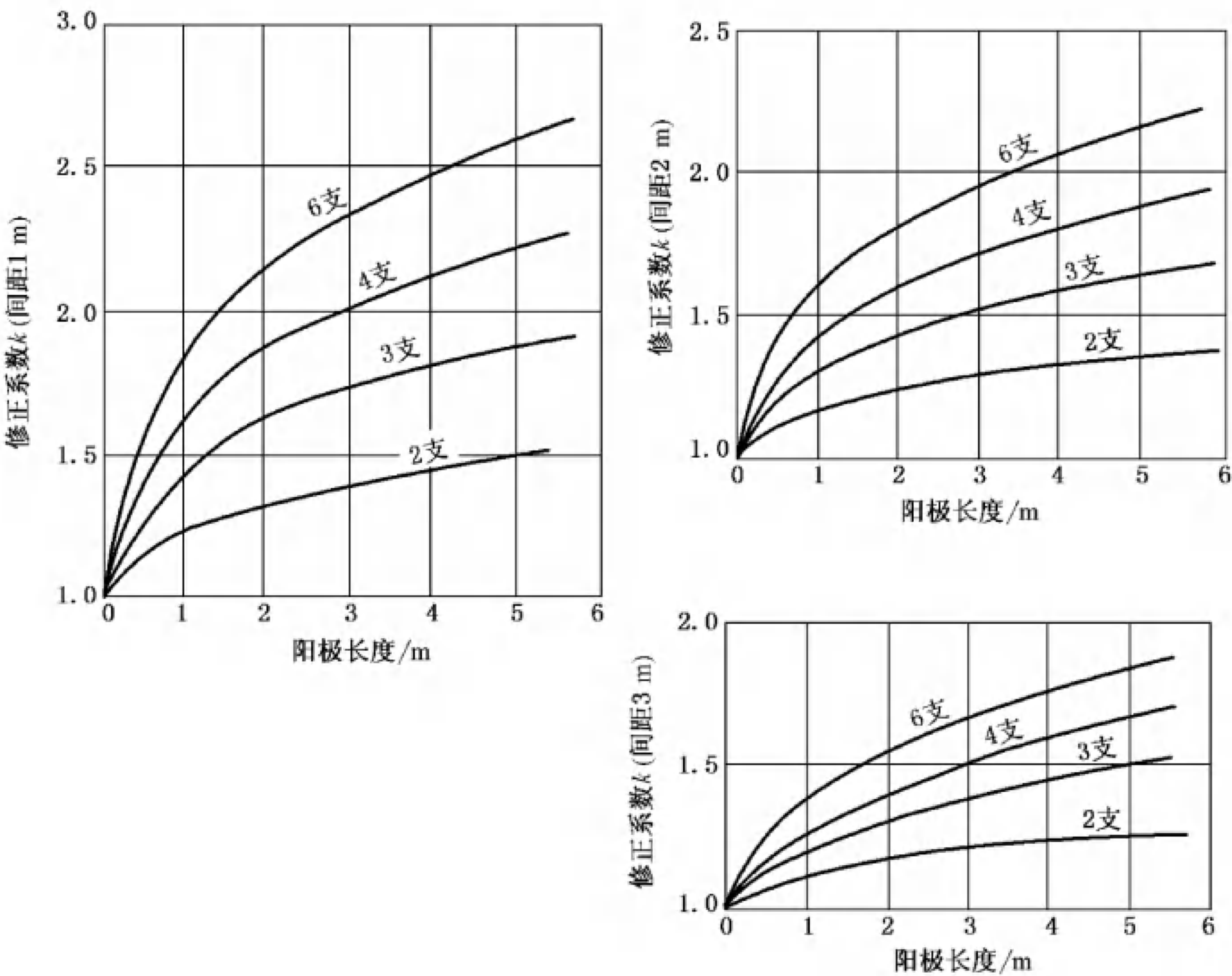
图 A.2 阳极接地电阻修正系数 k
