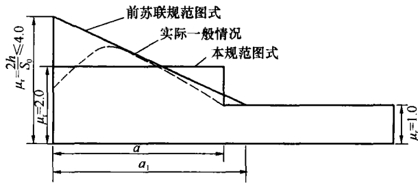
图 5 高低屋面处雪堆分布图示
