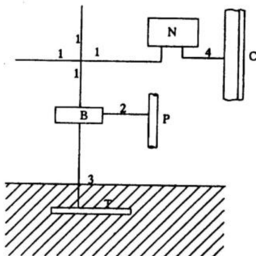
图 6 建筑物内总等电位联结图
