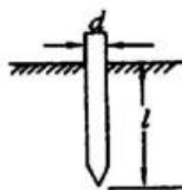
图 A1 垂直接地极的示意图
