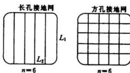
图 B1 接地网的形状
