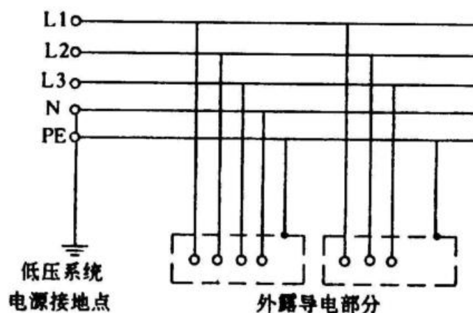
图 1 TN—S 系统, 整个系统的中性线与保护线是分开的
