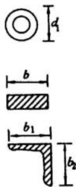
图 A2 几种型式钢材的计算用尺寸
